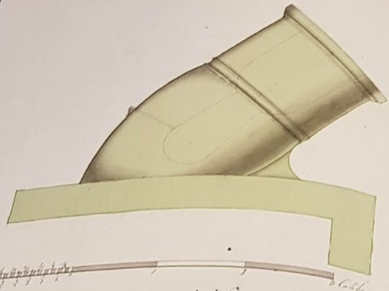
Tegning af en 100^{\text{m}} Metal Løe Morteer af Fr. 1/2 af rulle Størrelse
